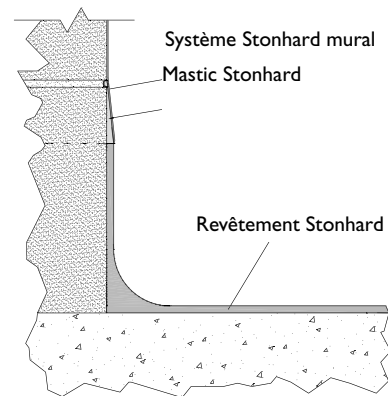
PLINTHE AVE FINITION DE HAUT DE PLINTHE
